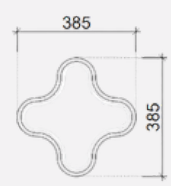
PLANTA
