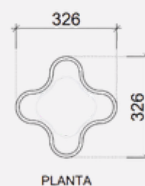
PLANTA
